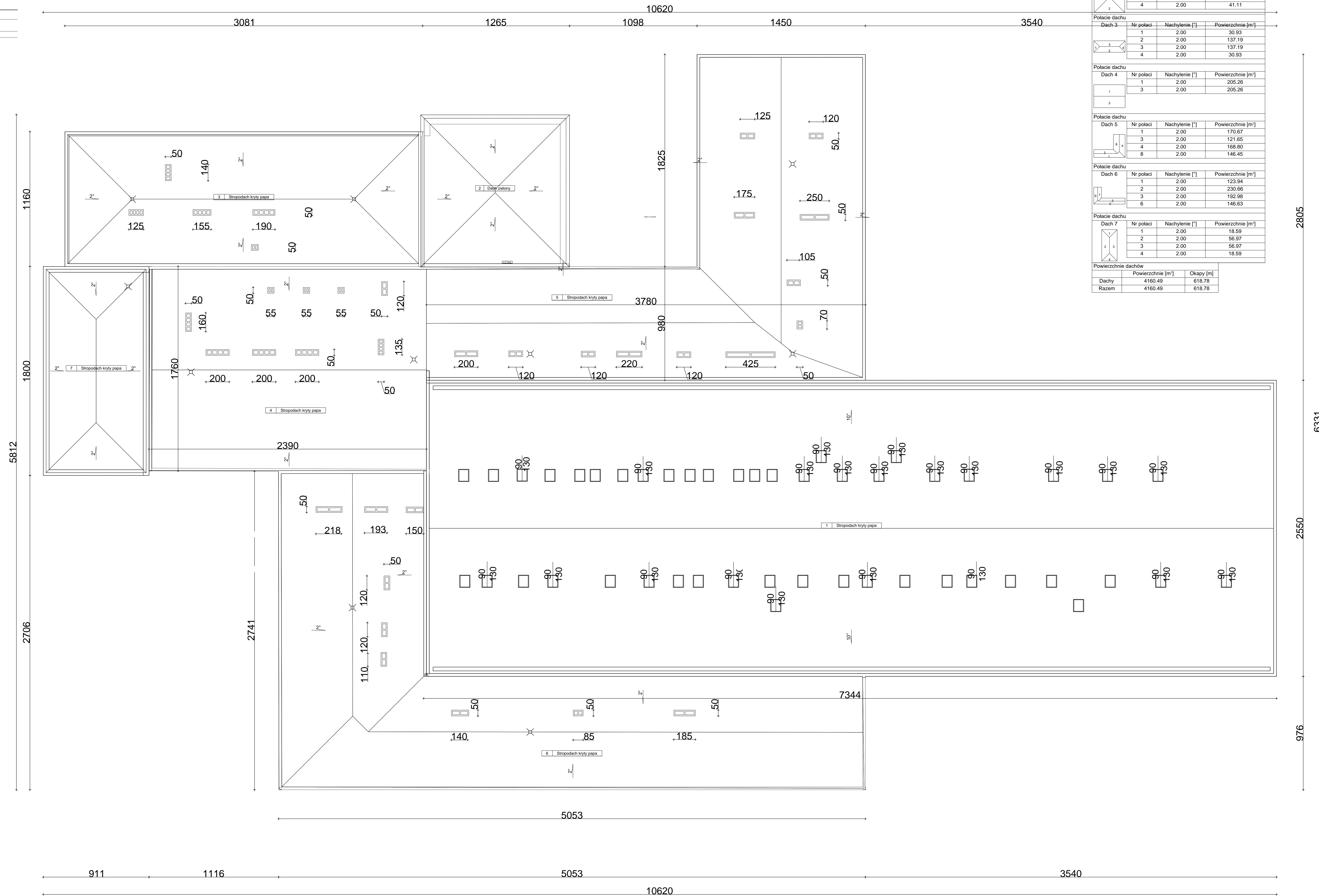
RZUT DACHU UL. OSTROBRAMSKA 101
